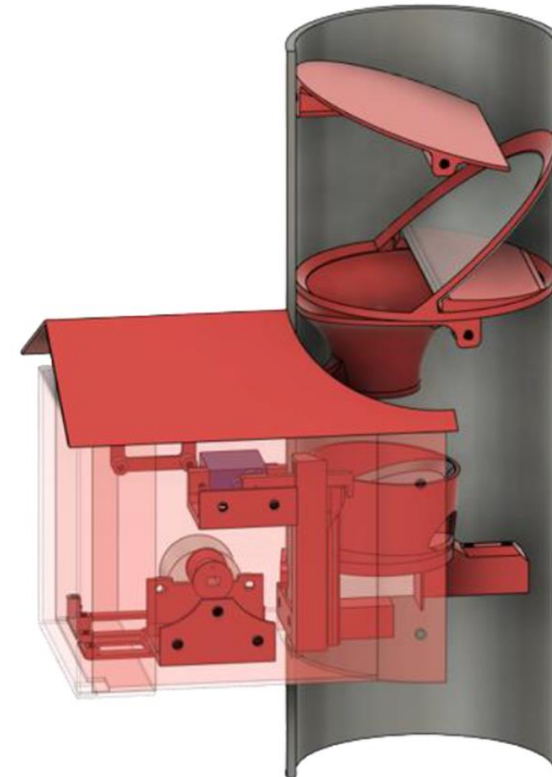
Figuur 2: Zandvanger eindproduct Fusion 360 ontwerp
