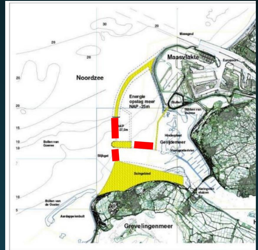
Figuur 26: Visualisatie locatie bouwputten
